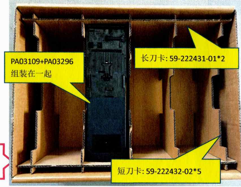
图二, 当 PA03109 内箱+PA03296 外箱组合出货时, 不用装透明袋, 折叠好内箱, 放置一块隔板和刀卡, 再将组装好的成品放入, 一箱四个。
